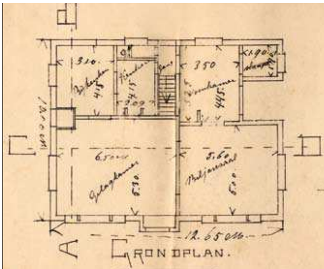
Details van de in het archief van Stad Hardenberg bewaard gebleven bouwtekening, anno 1918.
